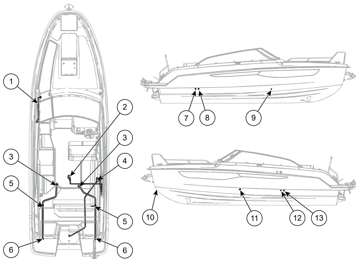
Kuva 9.1 Yamarin 80 DC pilssipumput ja tyhjennys
