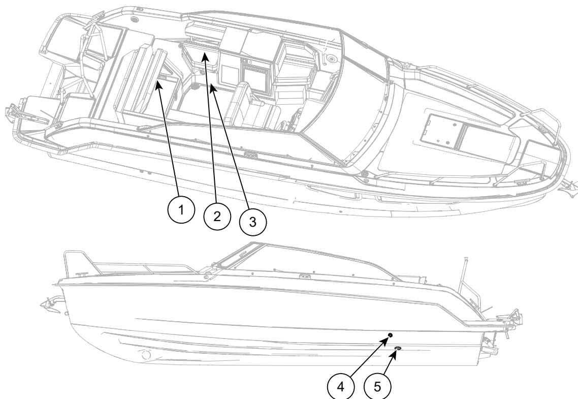
Kuva 11.3 Yamarin 80 DC:n ilmastointijärjestelmä
