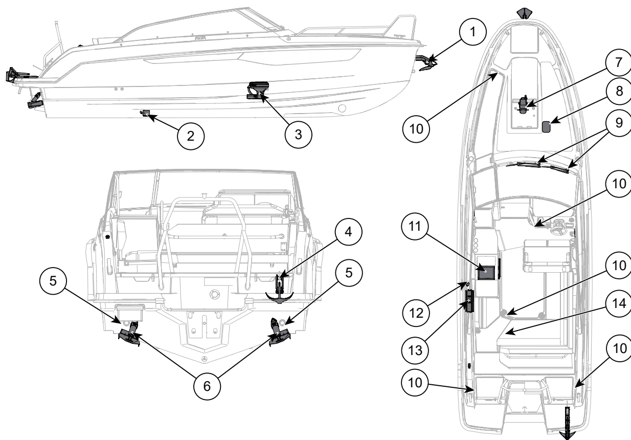
Kuva 8.2 Yamarin 80 DC sähkölaitteet
