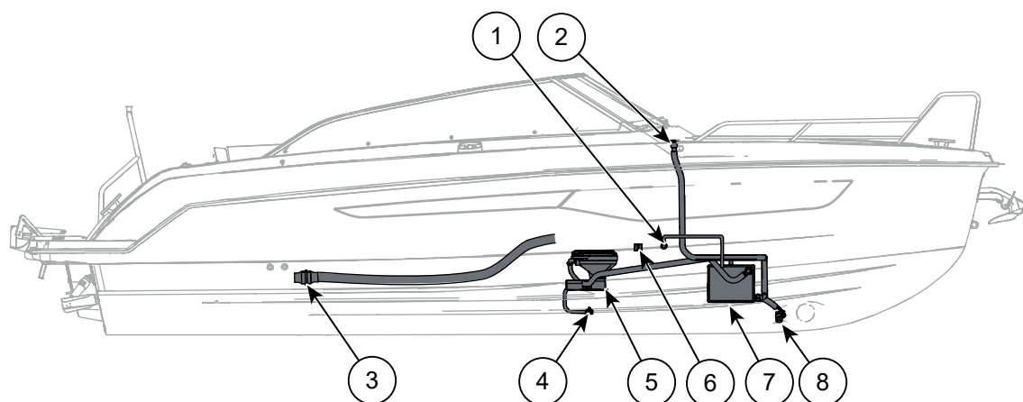
Kuva 11.1 Yamarin 80 DC septijärjestelmä
