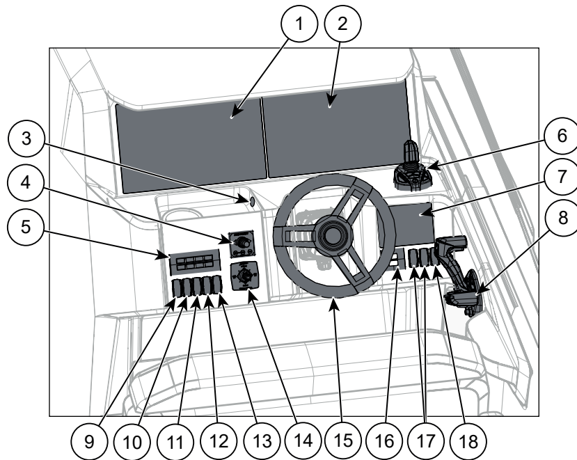
Kuva 5.1 Yamarin 80 DC ohjauspisteen hallintalaitteet
