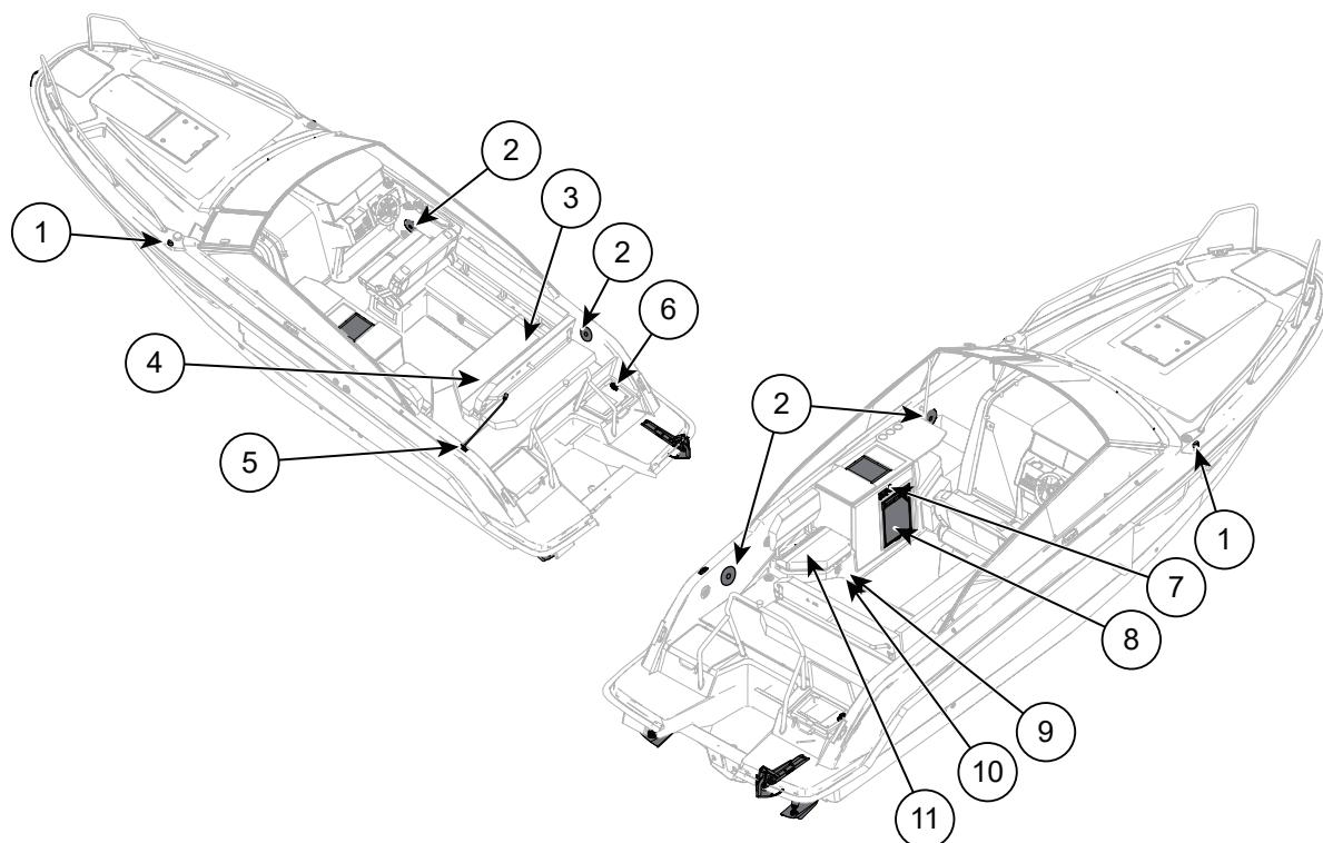
Kuva 8.3 Yamarin 80 DC sähkölaitteet
