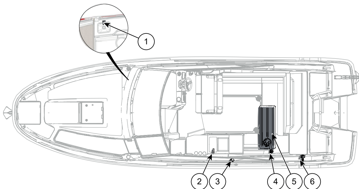
Kuva 10.1 Yamarin 80 DC makeavesijärjestelmä
