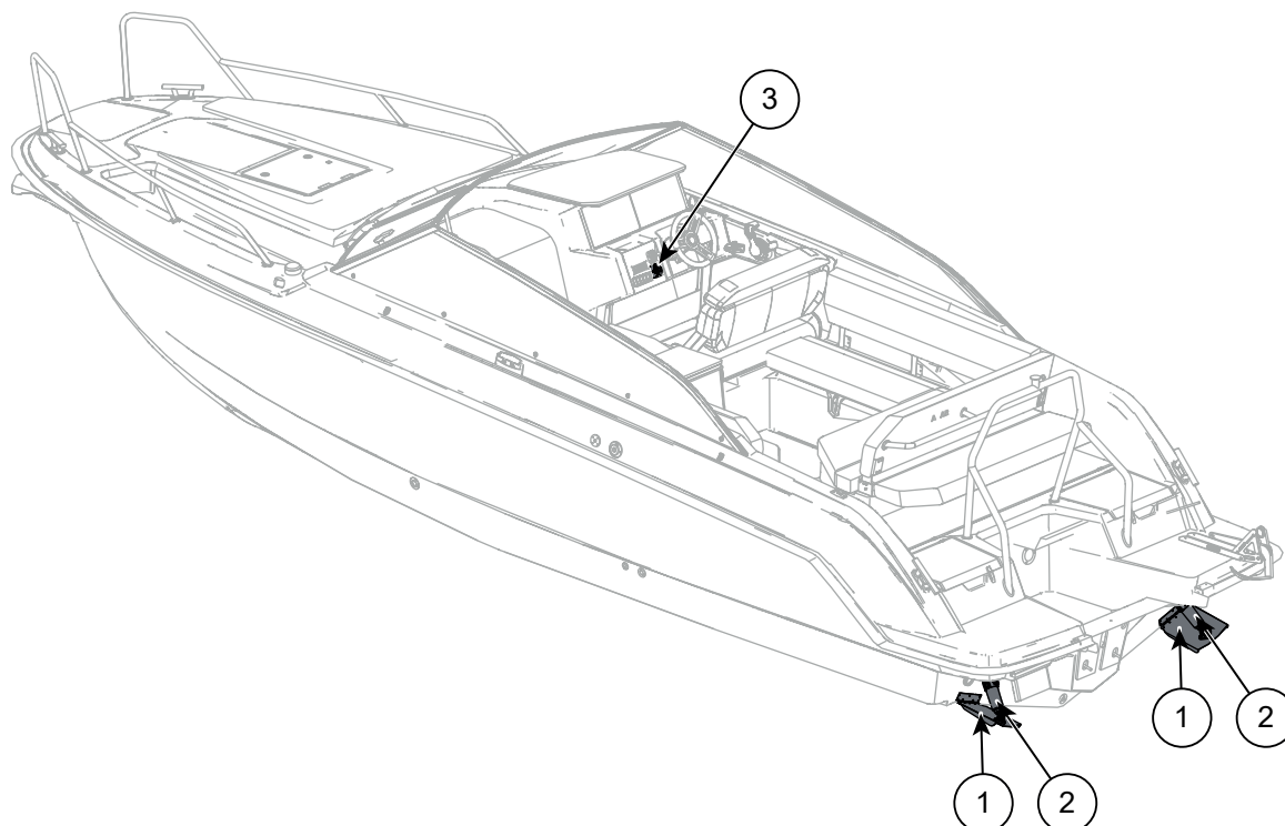
Kuva 5.10 Yamarin 80 DC trimmijärjestelmä
