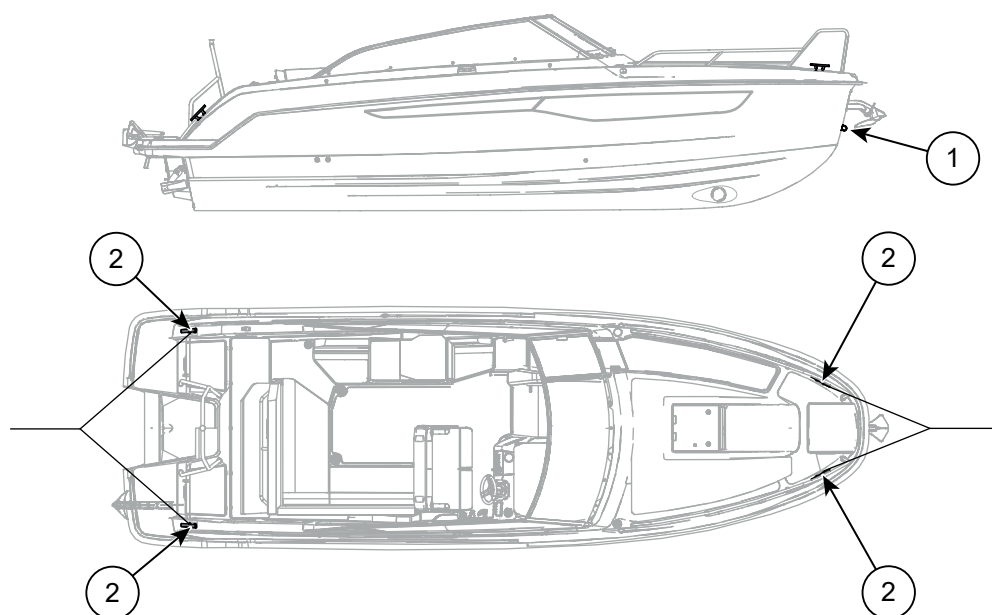
Kuva 5.11 Yamarin 80 DC kiinnitys- ja hinauspisteet
