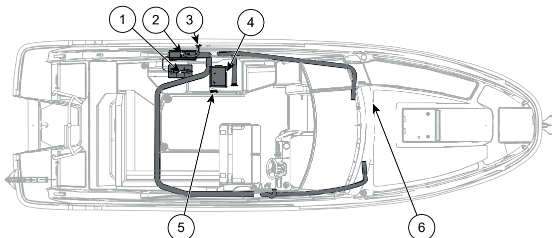
Kuva 6.2 Yamarin 80 DC polttoainekäyttöiset varusteet
